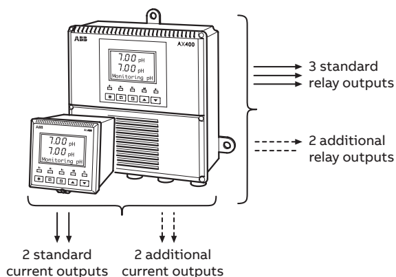
AX400 outputs
